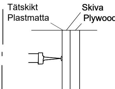
2. Applicera åldersbeständig tätningsmassa
