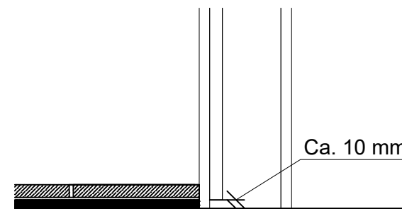
Avstånd konstruktionsplywood - undergolvet
