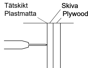
1. Markera skruvinfästning
