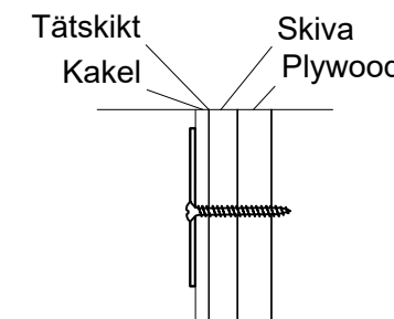
3. Montera med VVS-skruv
