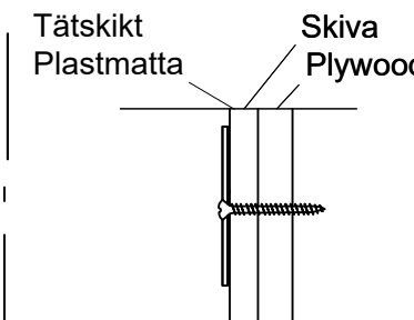
3. Montera med VVS-skruv
