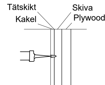
2. Applicera åldersbeständig tätningsmassa
